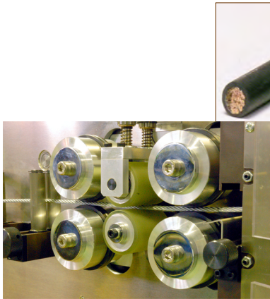
ロープワイヤー送り例 SA-382型
